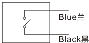
Output NO
